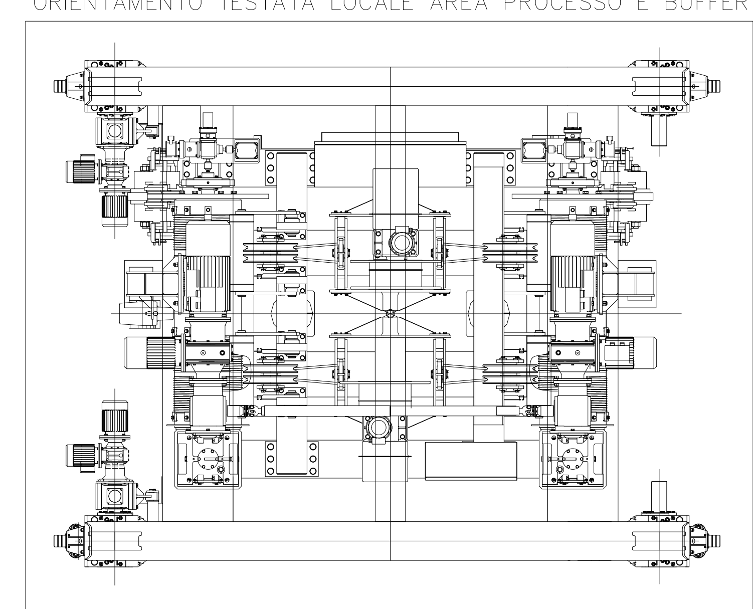
ORIENTAMENTO TESTATA LOCALE AREA PROCESSO E BUFFER
