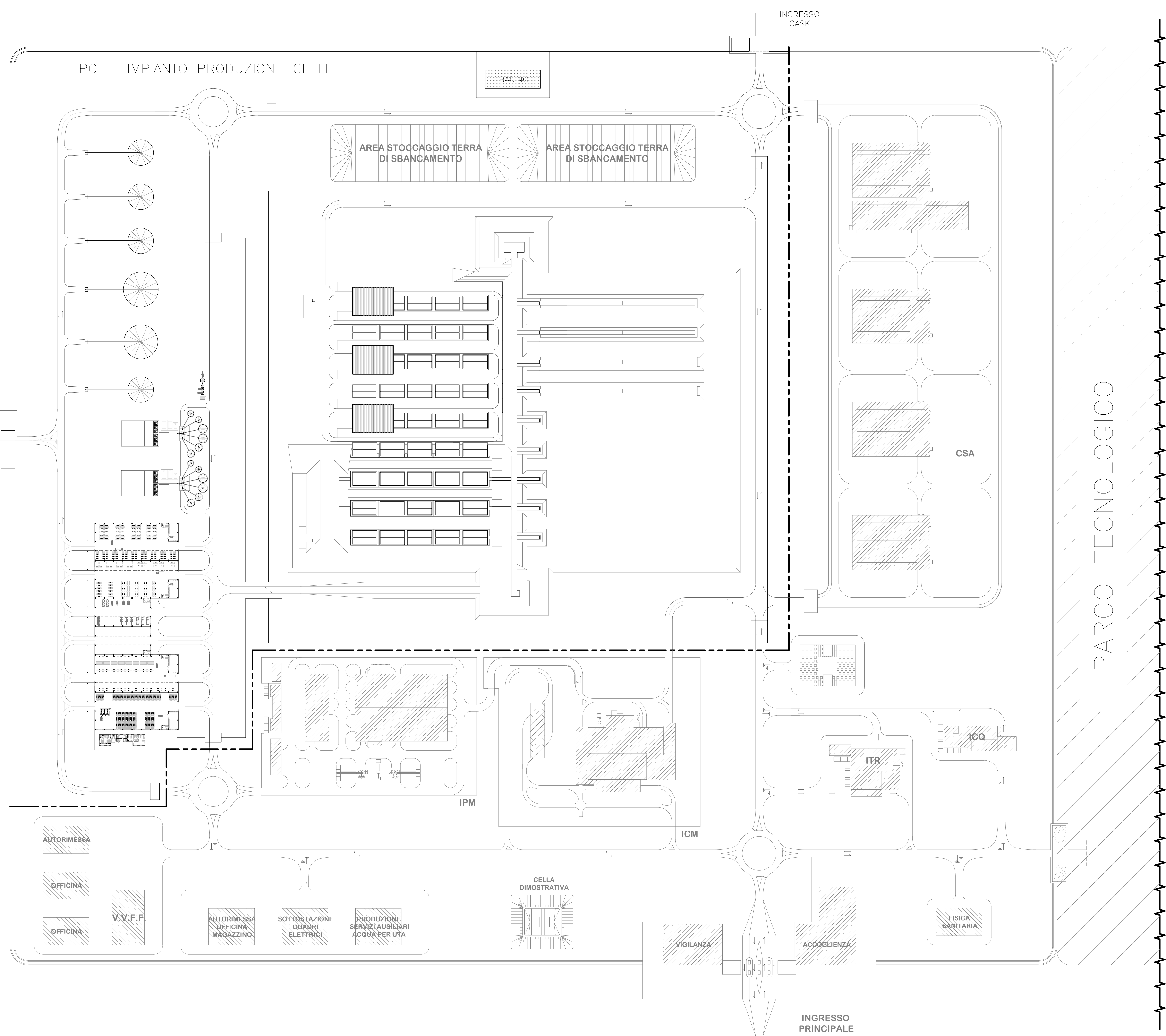
INQUADRAMENTO GENERALE IPC SCALA 1:2000
